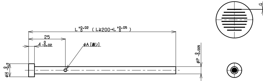
先端詳細図
